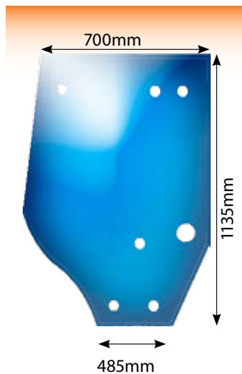
4938 Glass Case Maxxum Door Right Hand 7 Hole
