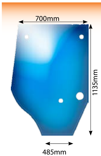
4974 Glass Case Maxxum Door Left Hand 4 Hole
