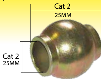
Top Link Ball CAT 2
